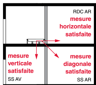
Banc d'essai avec dispositif d'essai et locaux de mesure. Le niveau d'exigence le plus élevé de l'isolation phonique est satisfait dans chaque sens de mesure.
