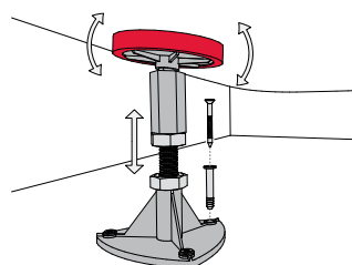
Pied de receveur avec mécanisme de tête articulée pour une grande précision d'ajustement et une grande stabilité (breveté et protection des modèles déposés)
