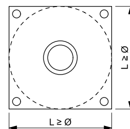
Plaque de montage avec goupille de serrage sur site Vue de dessus
