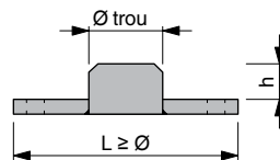
Plaque de montage avec goupille de serrage sur site Coupe
