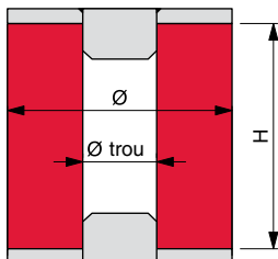
Pied de machine NIVO MA avec plaques de montage sur site Coupe
